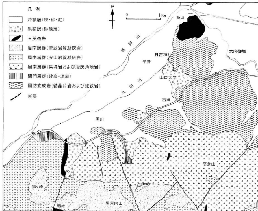
図1 平川地域の地質図
